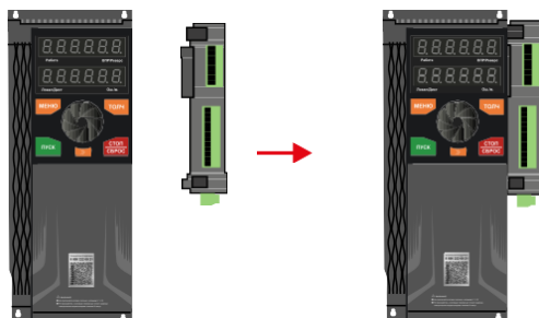
Рисунок 5.8 – Наружная установка модуля INMX-Ecard
