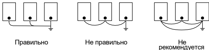
Рисунок 3.9 – Схематичное изображение образования петли с заземляющим проводом
