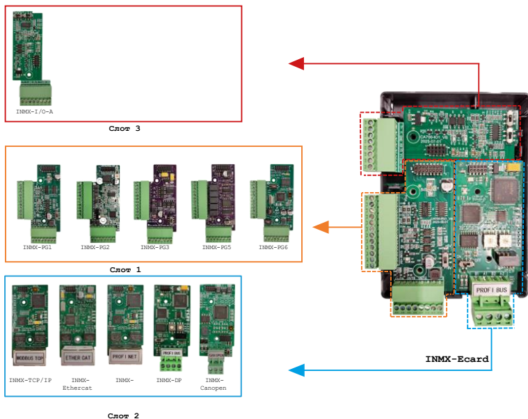
Рисунок 9.1 – Установка плат в модуль INMX-Ecard
